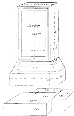
Fig. 24 Aufbau des Grabmonumentes von Fig. 25
