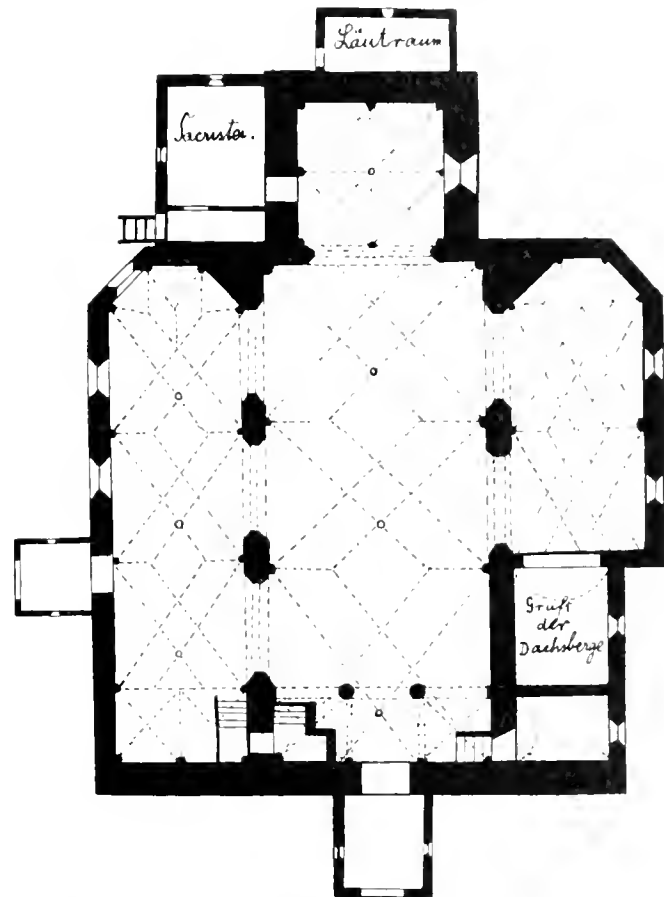
Fig. 53 Grundriß der Pfarrkirche zu Rapotenstein
