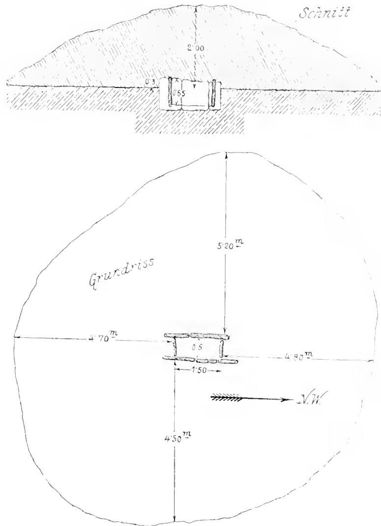
Fig. 132 Situation und Durchschnitt des Tumulusgrabes I auf dem Plateau Paravia bei Barbariga
