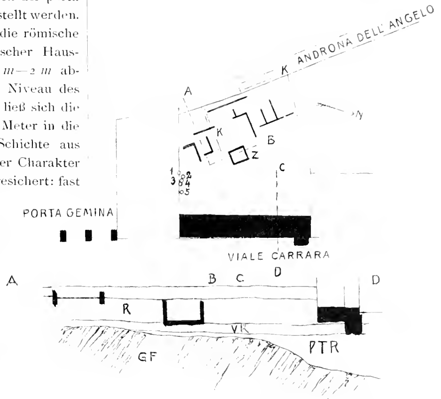
Fig. 67 Situation und Durchschnitt der Fundschichten am Bauplatz des Hauses viale Carrara n. 3. Maßstab 1:840
