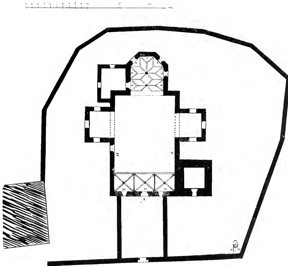
Fig. 48 Grundriß der zerstörten Kirche von Grad (Veldes)
